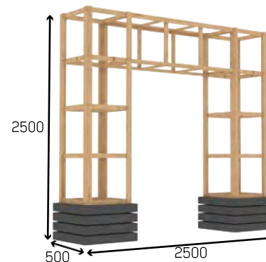
Арка
